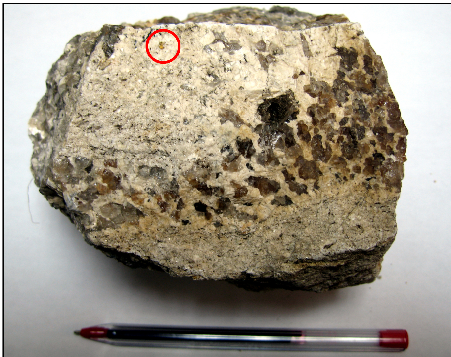
Trench Prospect : 992 g/t Au in quartz-feldspar pegmatite (Sample S657743)
