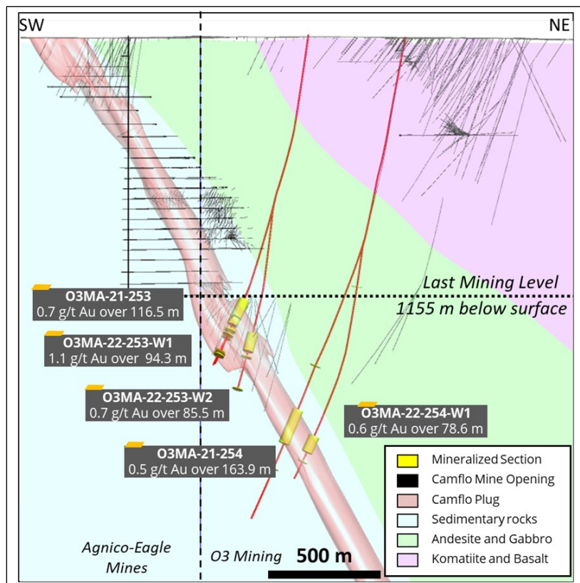
Figure 3 : Section transversale de l'extension Camflo
